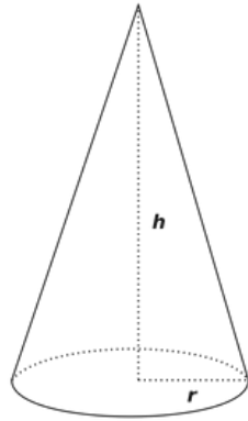
Cône
