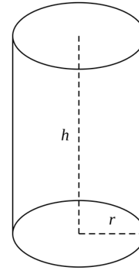
Cylindre
