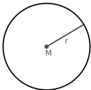
Cercle
